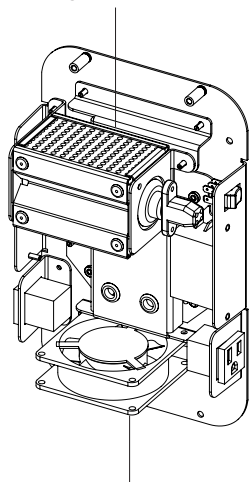
Assemblage de ventilateur
